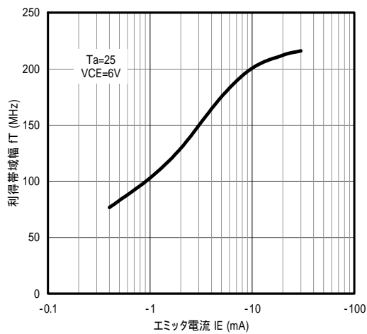
利得帯域幅 - エミッタ電流
