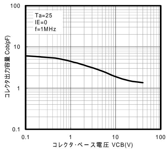
コレクタ出力容量 - コレクタ・ベース電圧特性
