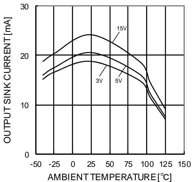
Figure 82. 出力シンク電流－温度特性 (OUT=VCC)
