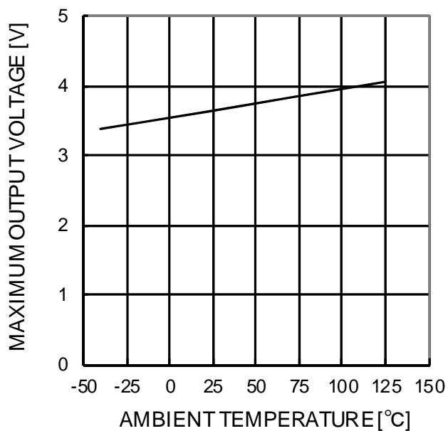
Figure 54. 最大出力電圧－温度特性 (VCC=5V, RL=2kΩ)
