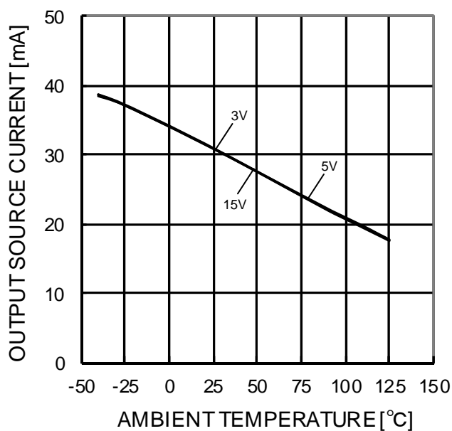
Figure 56. 出カソース電流－温度特性 (OUT=0V)
