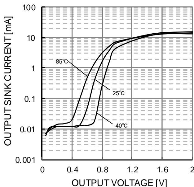
Figure 9. 出カシンク電流—出力電圧特性 (VCC=5V)
