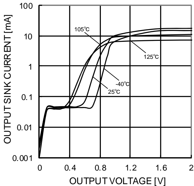
Figure 81. 出力シンク電流－出力電圧特性 (VCC=5V)
