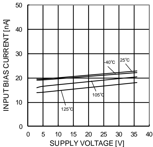
Figure 87. 入力バイアス電流-電源電圧特性 ( V_{ICM}=0V , OUT=1.4V )
