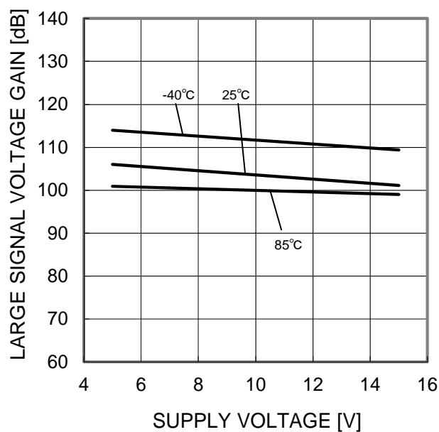
Figure 21. 大振幅電圧利得—電源電圧特性 (RL=2kΩ)
