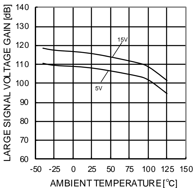
Figure 70. 大振幅電圧利得－温度特性 (RL=2kΩ)
