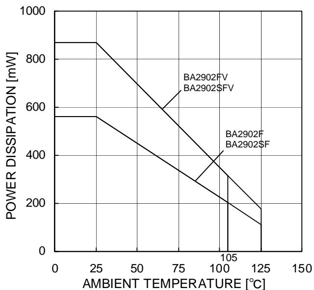
Figure 74. ディレーティングカーブ
