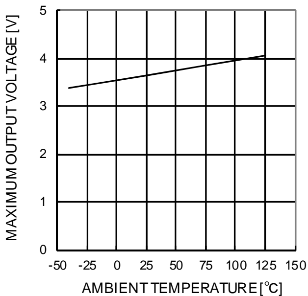
Figure 78. 最大出力電圧－温度特性 (VCC=5V, RL=2kΩ)
