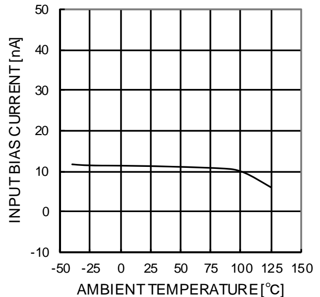
Figure 65. 入力バイアス電流-温度特性 ( VCC=30V , V_{ICM}=28V , OUT=1.4V )
