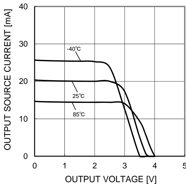
Figure 7. 出カソース電流—出力電圧特性 (VCC=5V)
