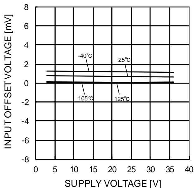
Figure 61. 入力オフセット電圧－電源電圧特性 (V ICM =0V, OUT=1.4V)
