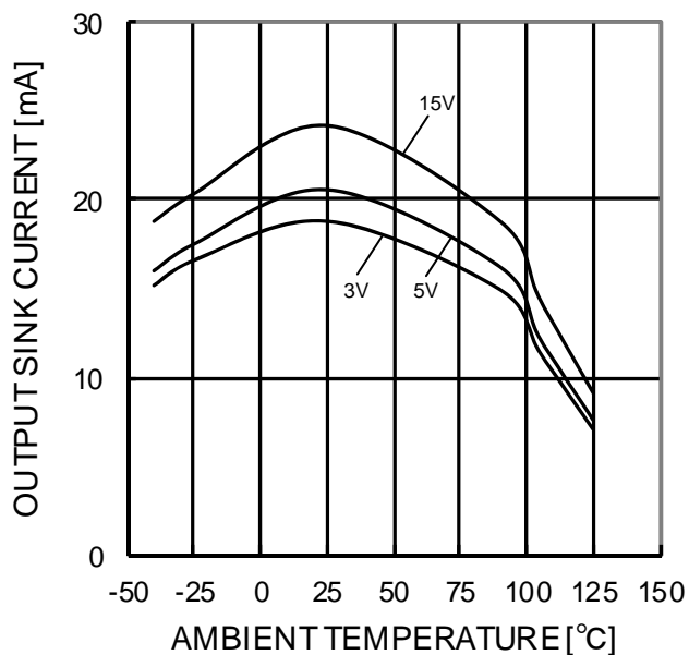
Figure 58. 出力シンク電流－温度特性 (OUT=VCC)
