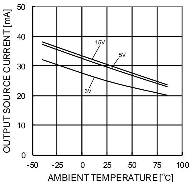
Figure 32. 出カソース電流－温度特性 (OUT=0V)
