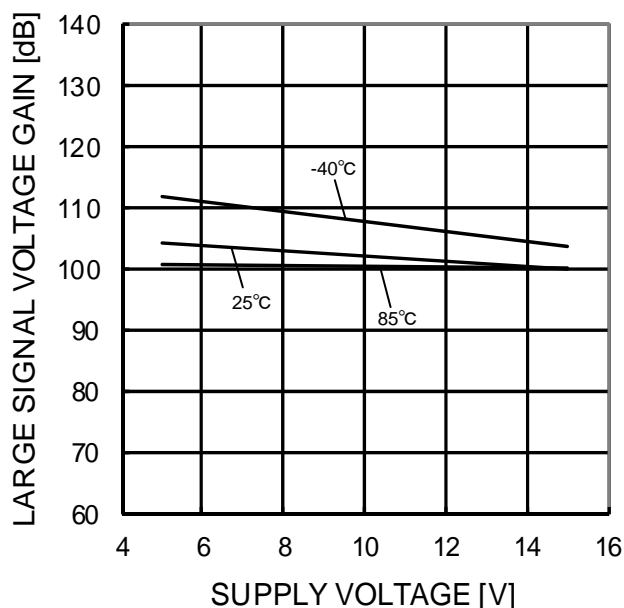
Figure 45. 大振幅電圧利得—電源電圧特性 (R L =2kΩ)
