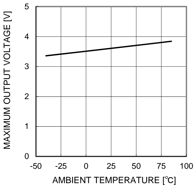
Figure 6. 最大出力電圧—温度特性 (VCC=5V,RL=2kΩ)
