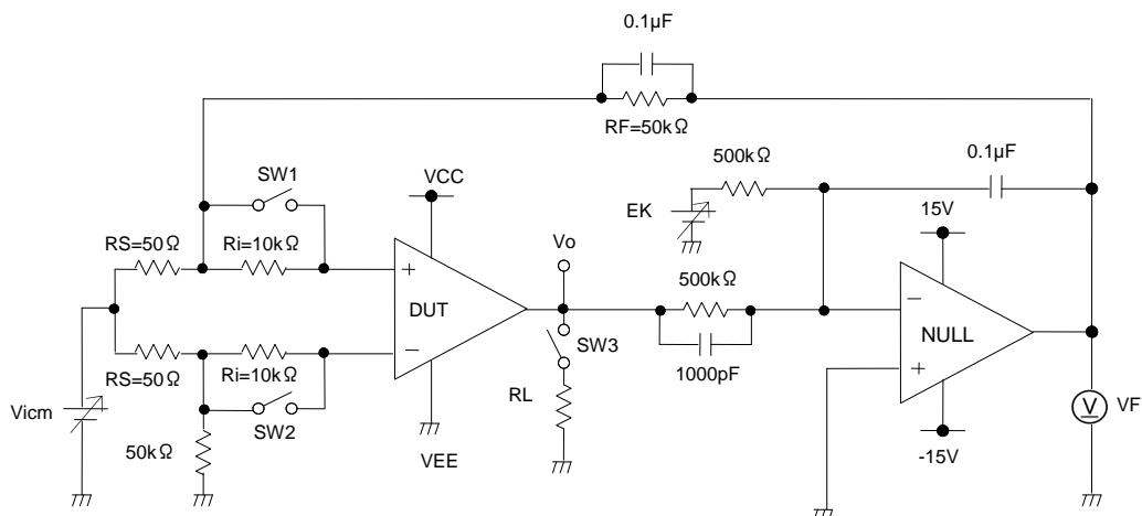
Figure 98. 測定回路 1 (1 チャンネルのみ)
