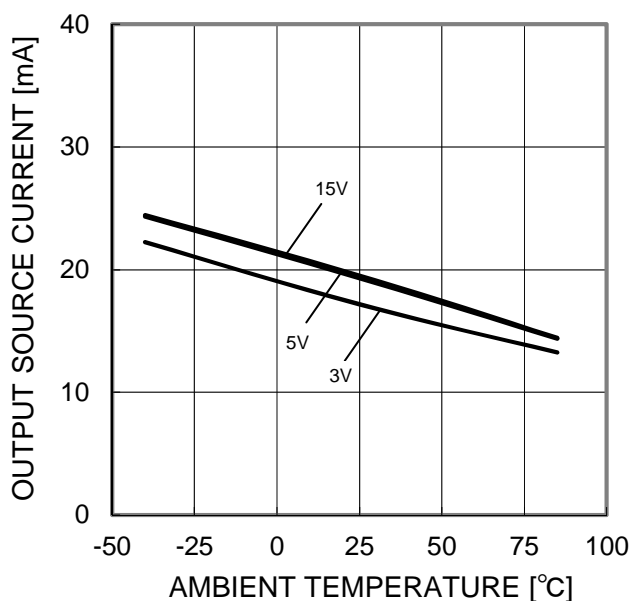
Figure 8. 出カソース電流—温度特性 (OUT=0V)
