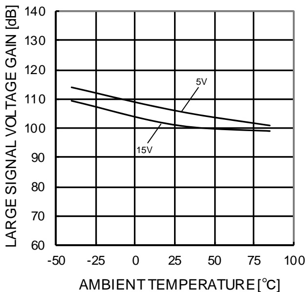
Figure 22. 大振幅電圧利得-温度特性 (RL=2kΩ)
