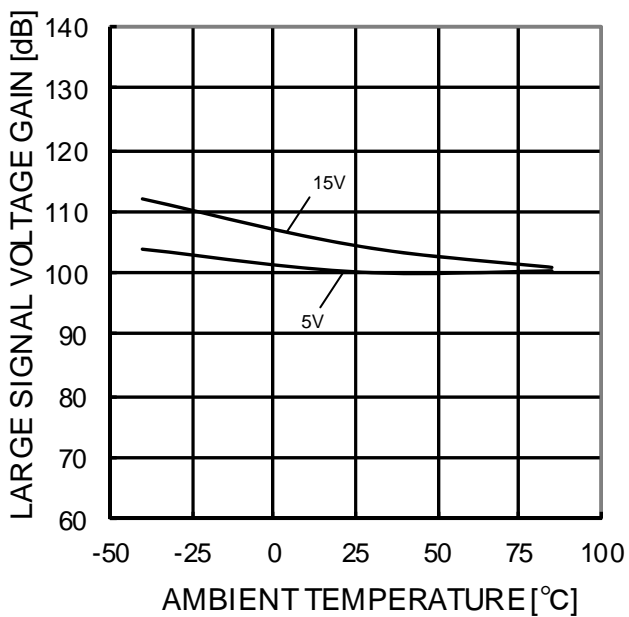
Figure 46. 大振幅電圧利得－温度特性 (RL=2kΩ)
