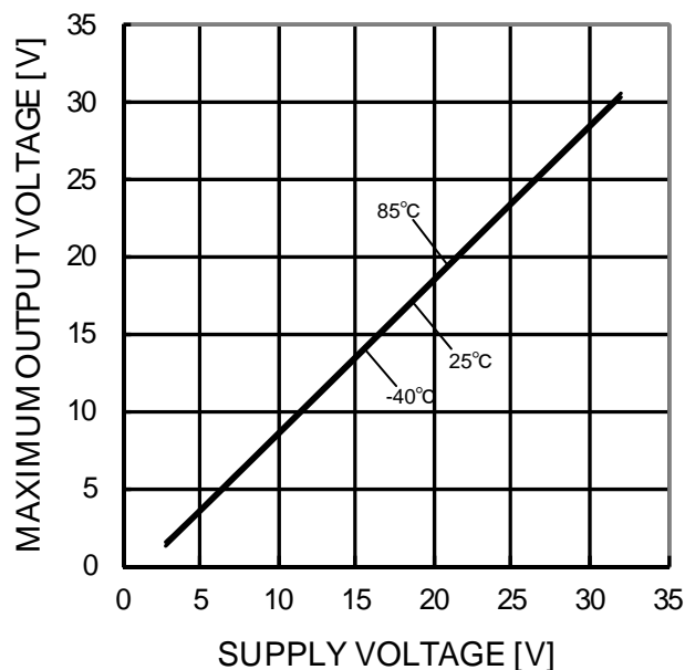
Figure 29. 出力電圧－電源電圧特性 (RL=10kΩ)
