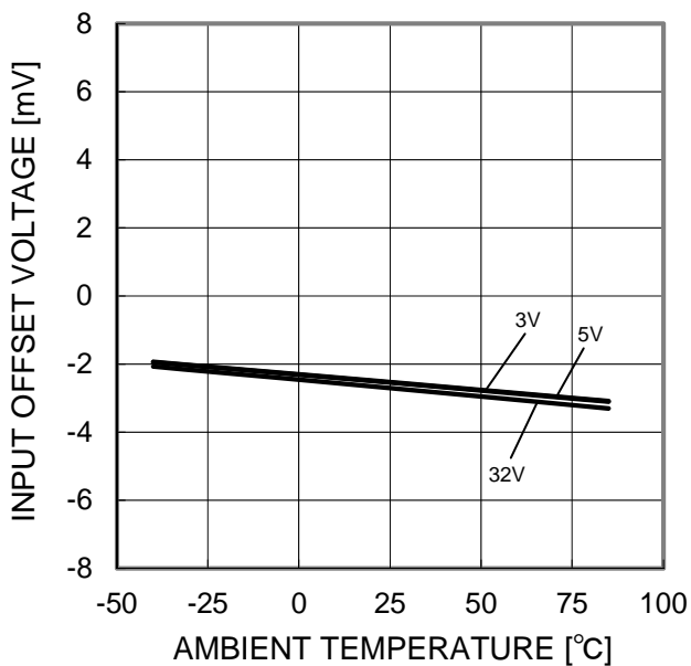
Figure 14. 入力オフセット電圧－温度特性 ( V_{ICM}=0V , OUT=1.4V )
