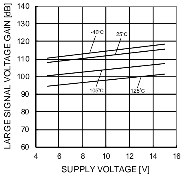
Figure 69. 大振幅電圧利得—電源電圧特性 (RL=2kΩ)
