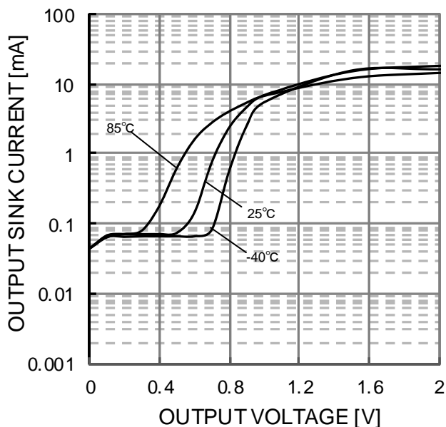
Figure 33. 出カシンク電流－出力電圧特性 (VCC=5V)
