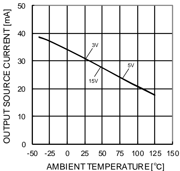
Figure 80. 出力ソース電流－温度特性 (OUT=0V)
