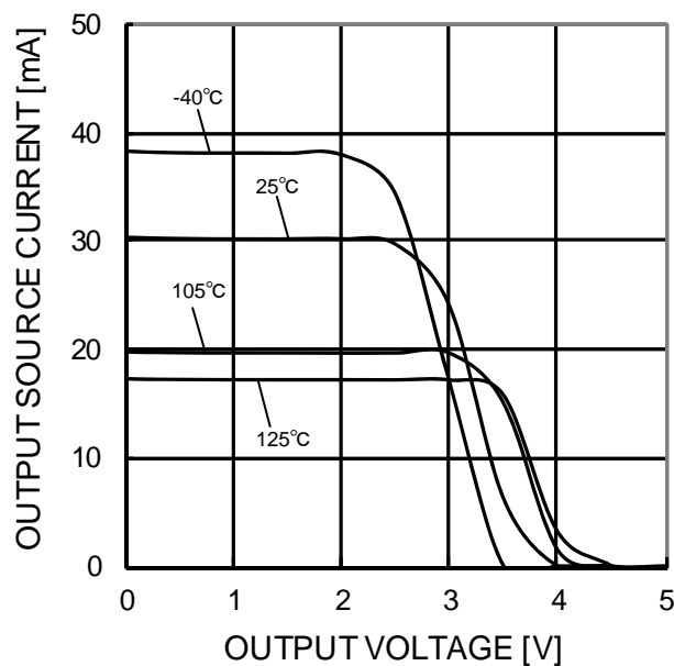
Figure 55. 出カソース電流－出力電圧特性 (VCC=5V)
