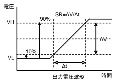
Figure 100. スルーレート測定時 入出力波形
