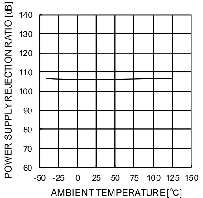
Figure 97. 電源電圧除去比－温度特性
