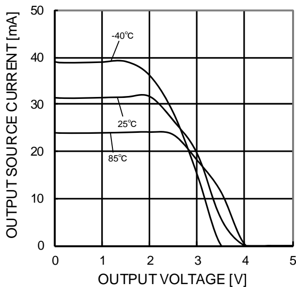
Figure 31. 出カソース電流－出力電圧特性 (VCC=5V)
