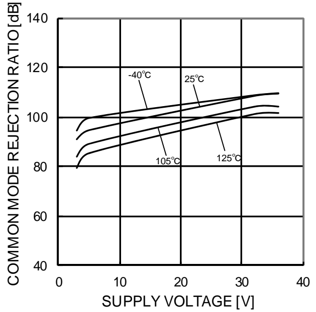
Figure 95. 同相信号除去比－電源電圧特性
