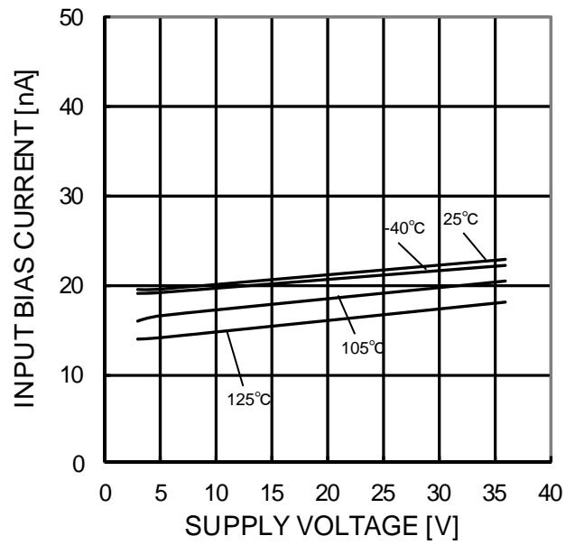
Figure 63. 入力バイアス電流-電源電圧特性 ( V_{ICM}=0V , OUT=1.4V )
