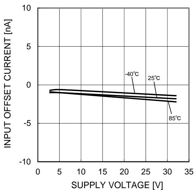
Figure 19. 入力オフセット電流—電源電圧特性 (VICM=0V, OUT=1.4V)
