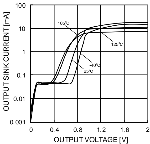
Figure 57. 出カシンク電流－出力電圧特性 (VCC=5V)
