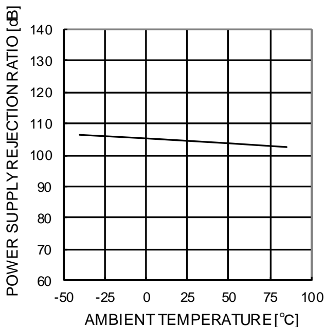
Figure 25. 電源電圧除去比-温度特性
