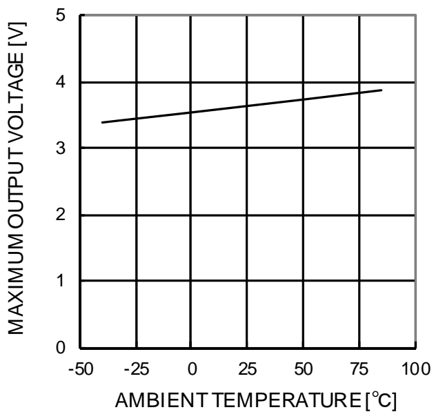
Figure 30. 最大出力電圧－温度特性 (VCC=5V, RL=2kΩ)
