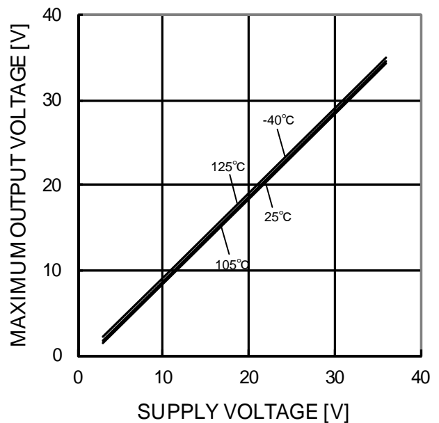
Figure 53. 出力電圧－電源電圧特性 (RL=10kΩ)
