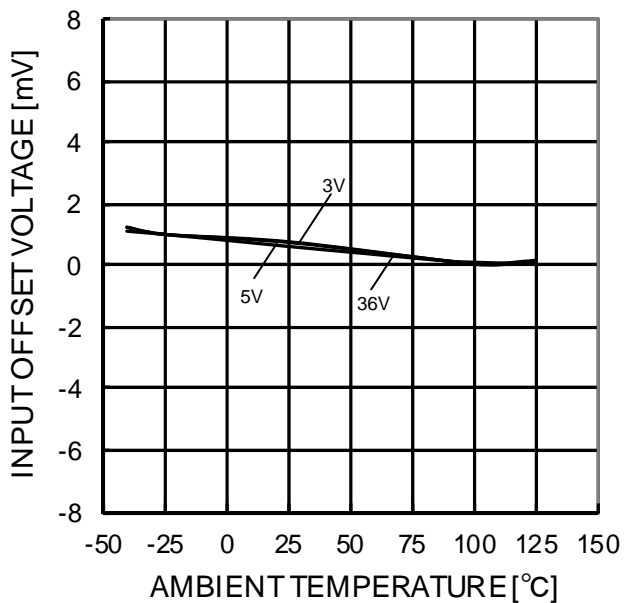
Figure 86. 入力オフセット電圧-温度特性 ( V_{ICM}=0V , OUT=1.4V )
