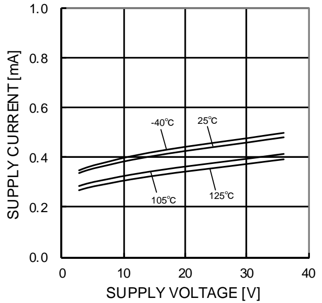
Figure 51. 回路電流－電源電圧特性
