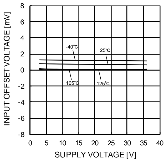
Figure 85. 入力オフセット電圧－電源電圧特性 (V ICM =0V, OUT=1.4V)
