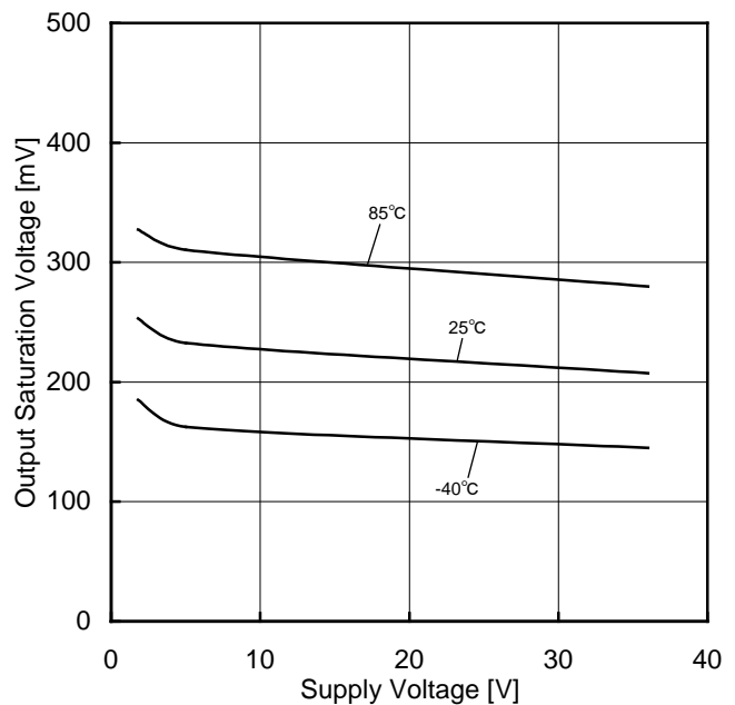
Figure 48. 出力飽和電圧—電源電圧特性 (I SINK =4mA)
