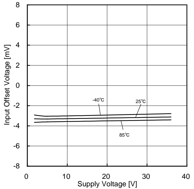
Figure 52. 入力オフセット電圧－電源電圧特性
