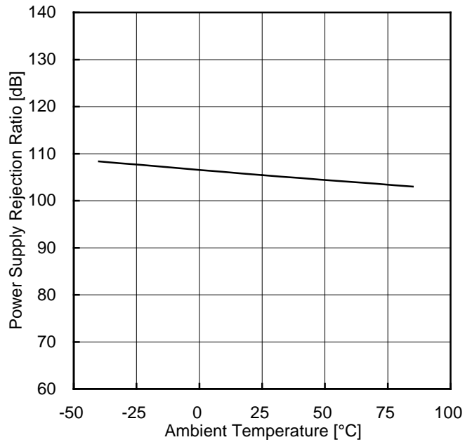
Figure 62. 電源電圧除去比-温度特性
