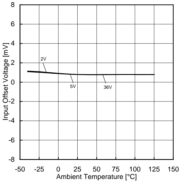
Figure 96. 入力オフセット電圧-温度特性
