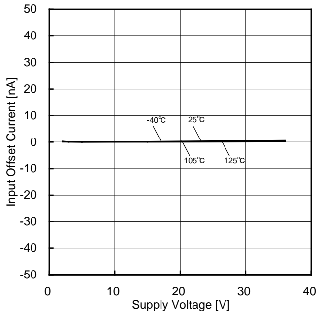
Figure 99. 入力オフセット電流-電源電圧特性
