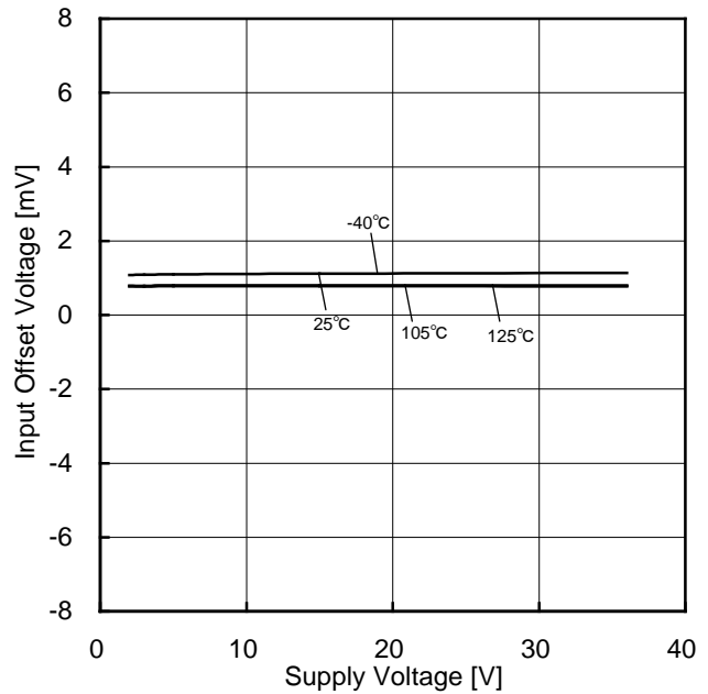
Figure 72. 入力オフセット電圧-電源電圧特性
