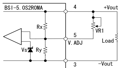
内部回路図 (図8)
