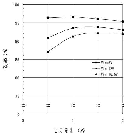
効率特性(図11)
