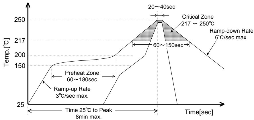
図 20 リフロー温度プロファイル（無鉛品）
