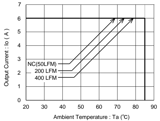
図 13 BST04M-0.7S06PDM (Vin=5.0V, Vo=1.8V)
