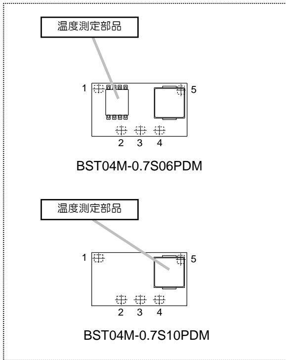
図 10 温度測定ポイント
