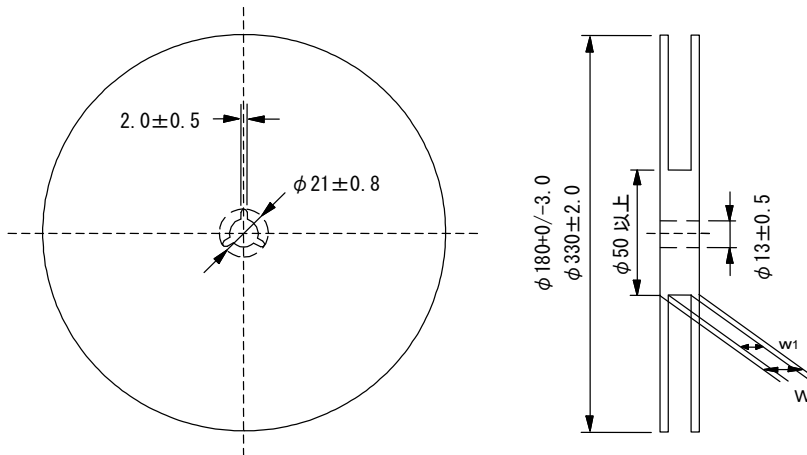
図2 リール寸法
