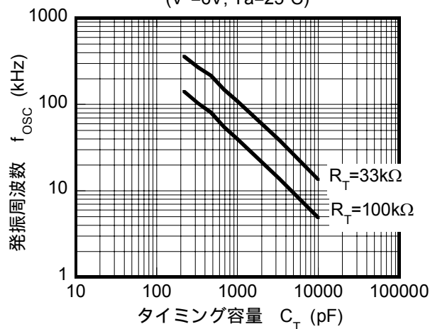
発振周波数対タイミング容量特性例
