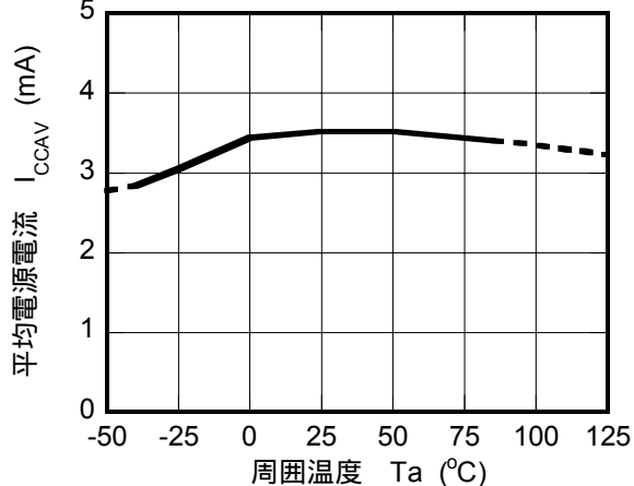
平均電源電流温度特性例
