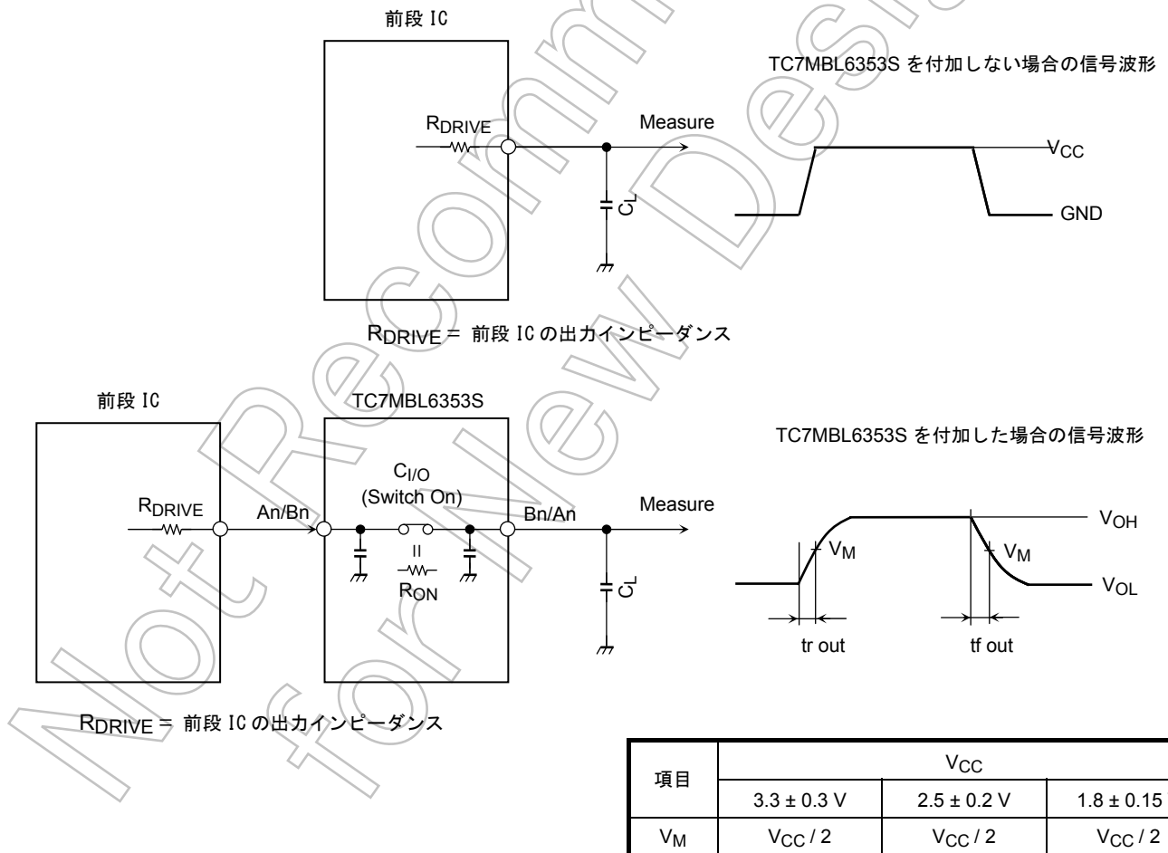
図 4 算出回路
