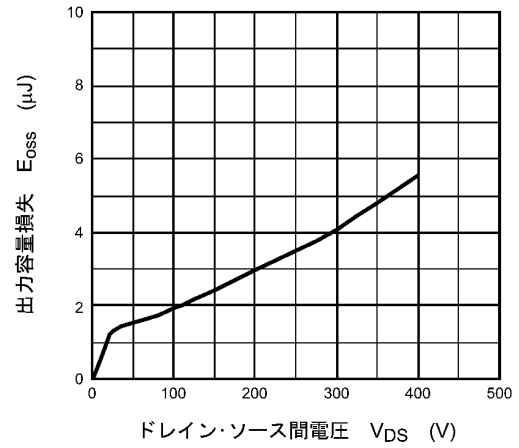
図 8.10 E_{oss} - V_{DS}
