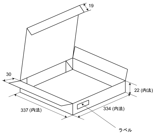
図 16.4.1 1リール入り梱包箱 (unit: mm)
