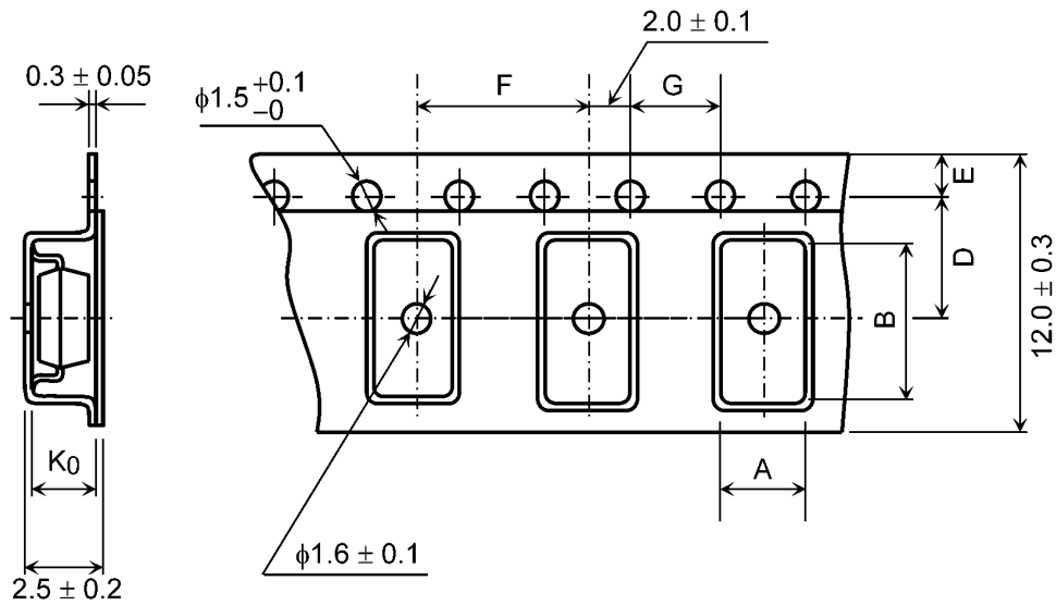
図 16.3.5.1 テープ形状
