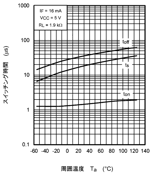
図 11.15 スイッチング時間 - T_a
