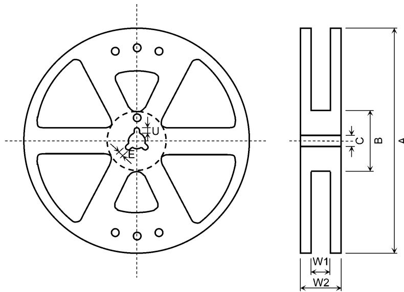
図 16.3.6.1 リール形状
