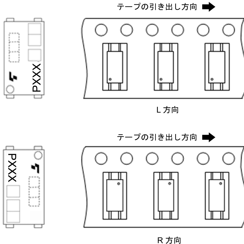
図 16.3.1.1 凹み角穴内の製品の向き
