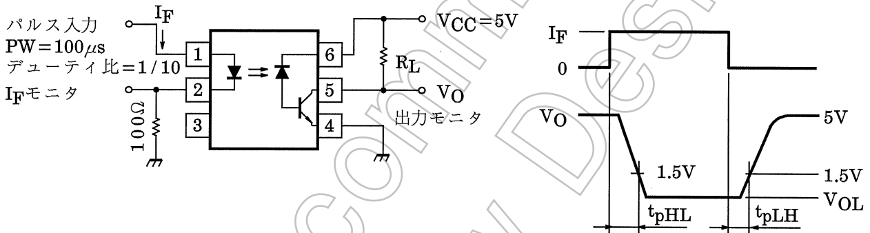
図 1 伝搬遅延時間測定回路、波形
