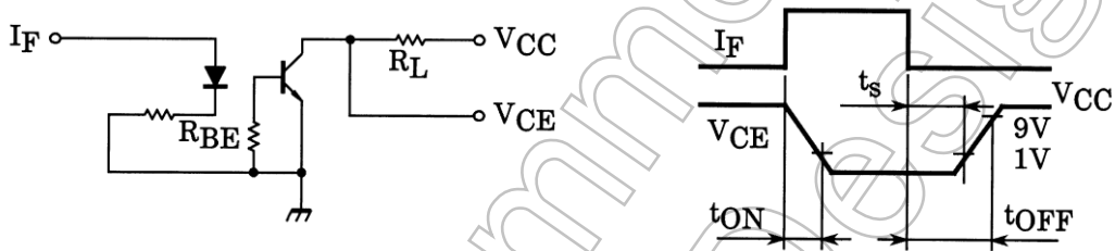
図 1: スwitchング時間測定回路
