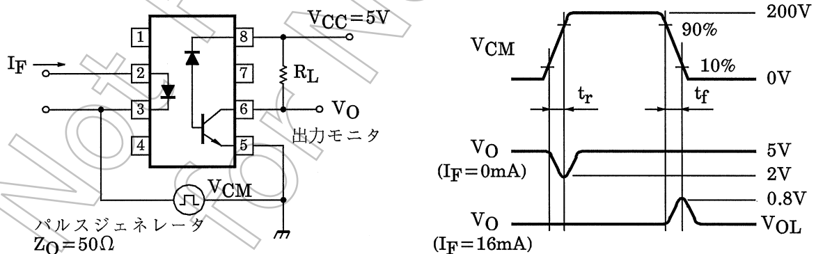
図 2. コモンモードノイズ除去電圧測定回路、波形
